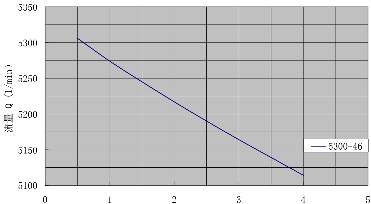
SN5300性能曲线 转速:1450r/min 粘度:75mm 2 /s
